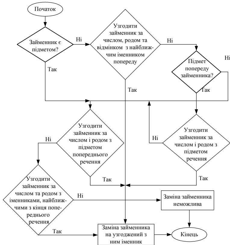
РИС. 2. Блок-схема алгоритму заміни займенників
