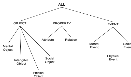
Рис.4. Верхний уровень онтологии Mikrokosmos
